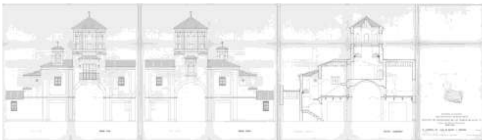
Link 12. Puerta de Loja, alzados y sección longitudinal; proyecto de 1985. (Archivo Histórico Provincial de Granada. Sección COAr. Signatura P-08).
