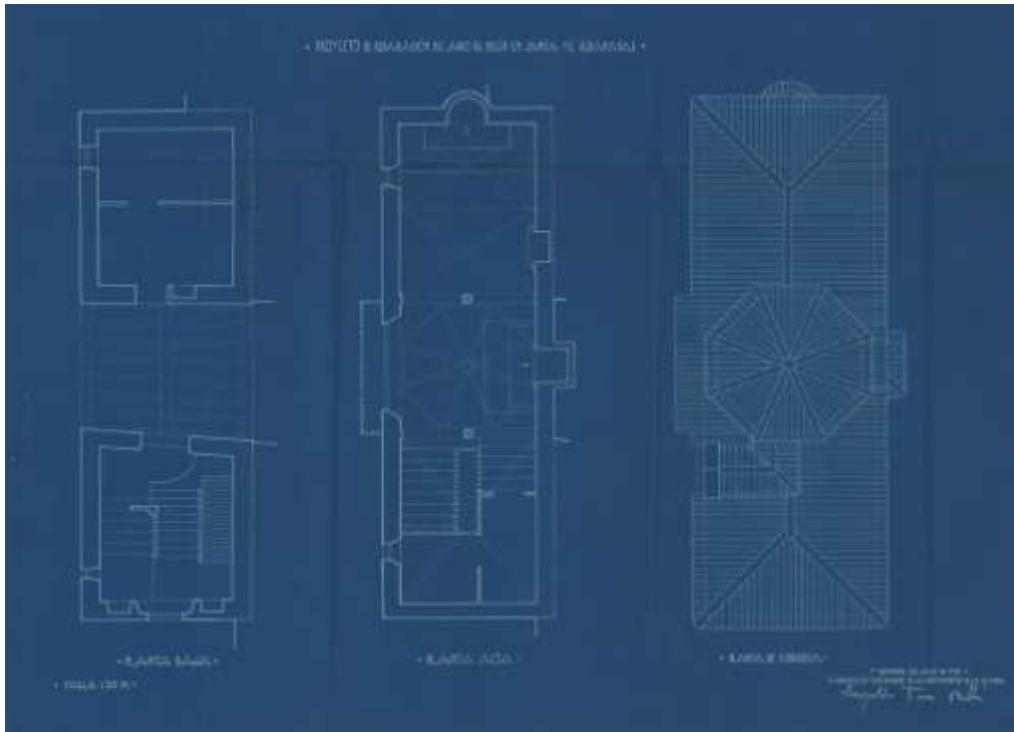
Link 05. Copia al ferroprusiato del plano original recogido por el proyecto de reparación del Arco de Belén en Santa Fe (Granada) de 1931, firmado por Torres Balbás (Archivo General de la Administración. Signatura (5) 14.2.; top. 31/04824).
