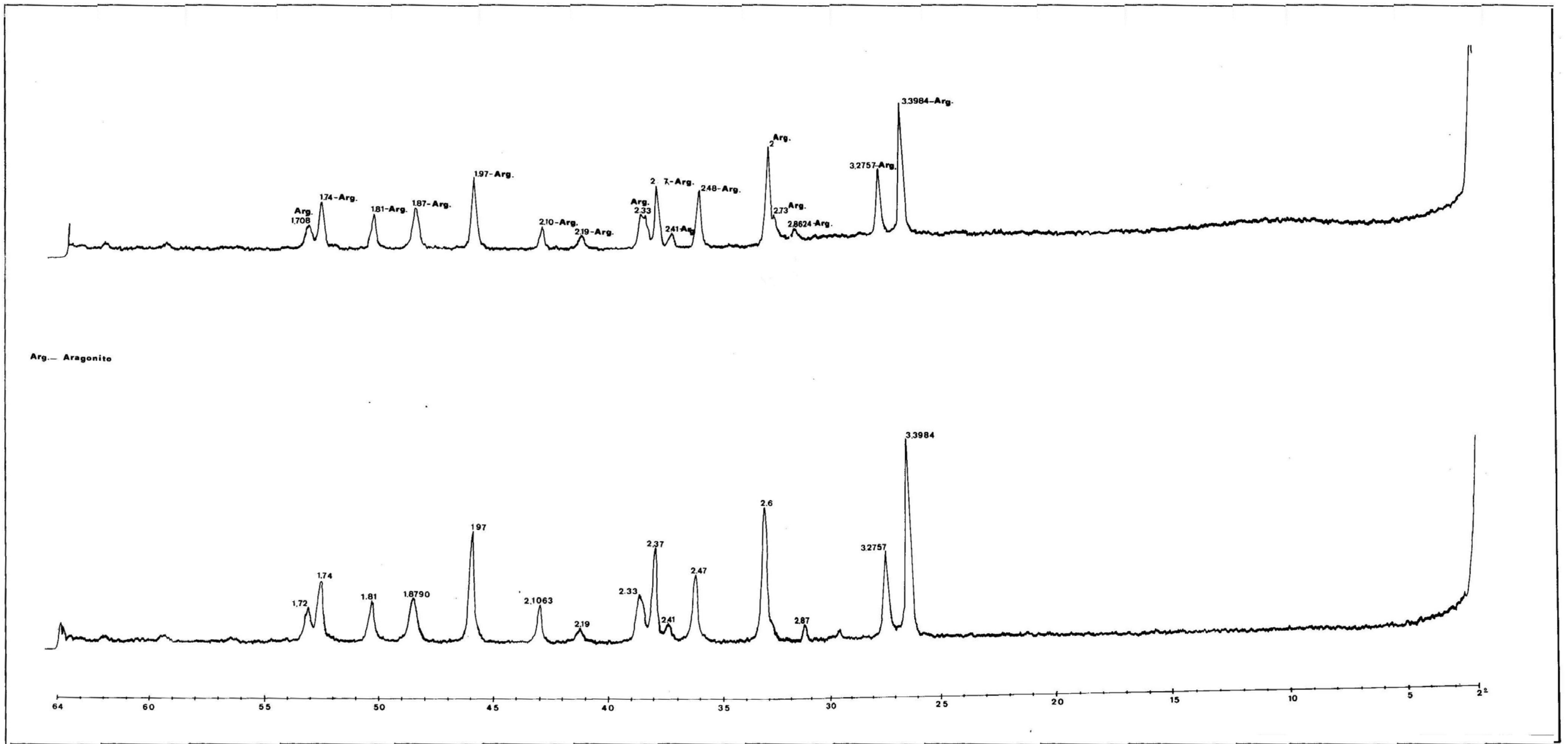
Fig. 3.—Diagramas obtenidos del análisis mediante Difracción de Rayos X de dos pequeñas cuentas discoidales.
