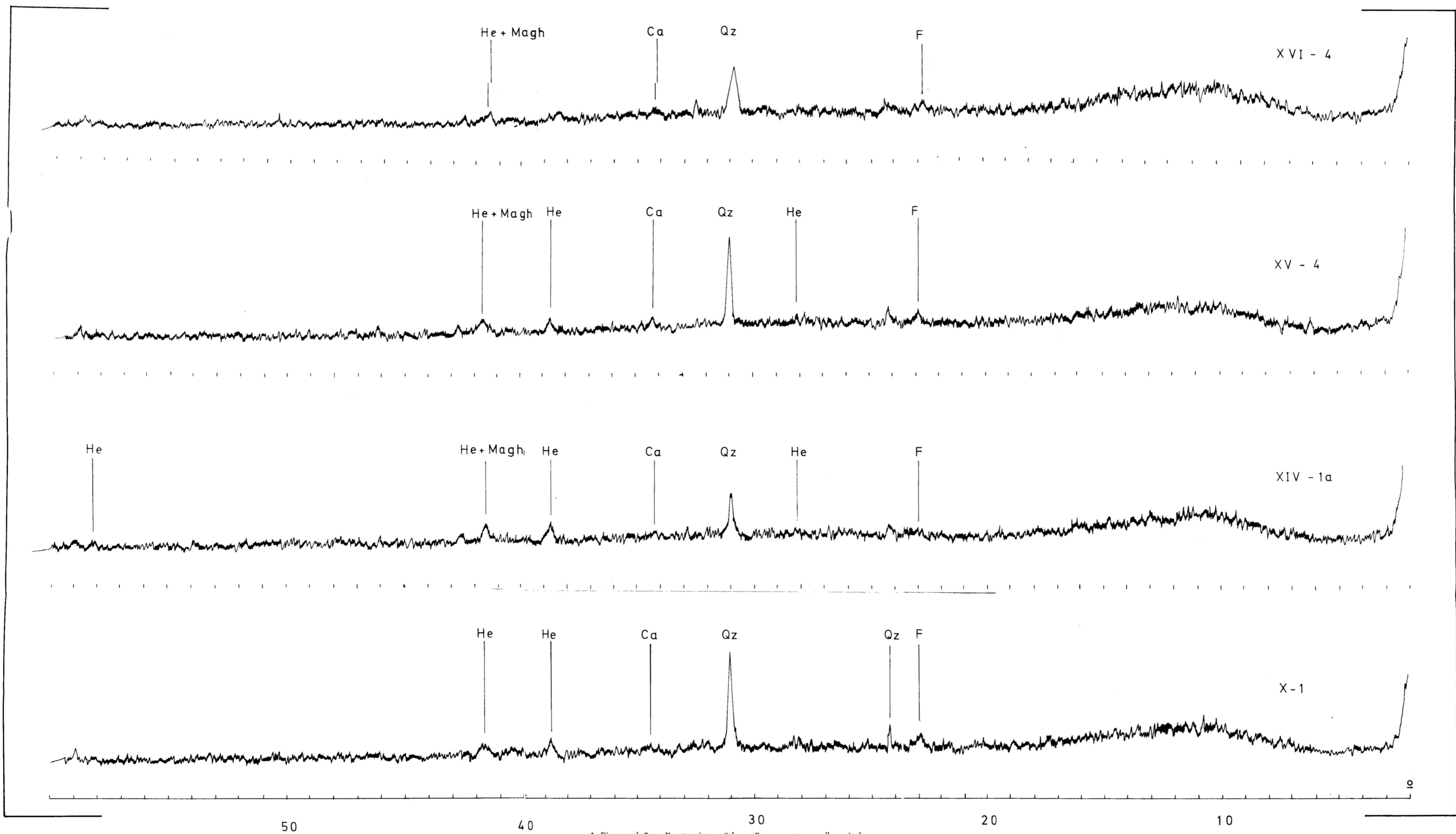
A.- Diagramas de Rayos X pertenecientes a "almagras" que presentan una adherencia clara.
