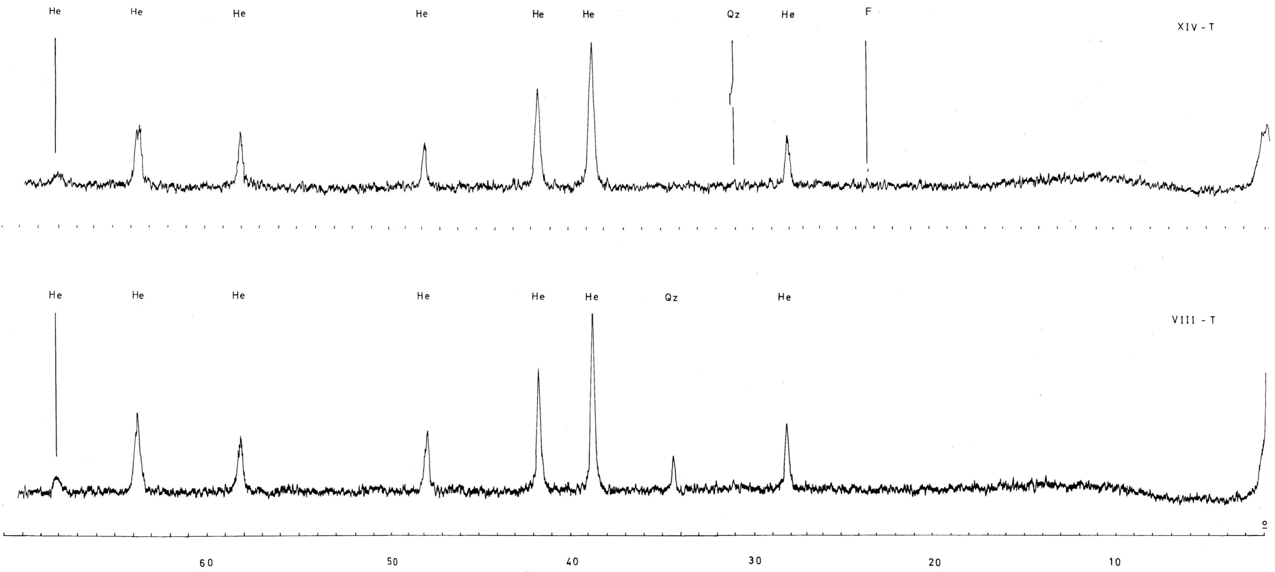
Fig. 3. Diagramas de Rayos X pertenecientes a dos trozos de mineral de hierro aparecidos en los estratos VIII y XIV respectivamente de la estratigrafía general de la "Cueva de la Carigüela".
