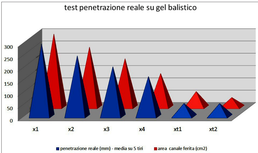
Fig. 9.—Test su gel balistico: comparazione delle diverse penetrazioni e dimensioni del canale di taglio in funzione della morfologia della cuspidè (freccè della stessa massa e velocità).
