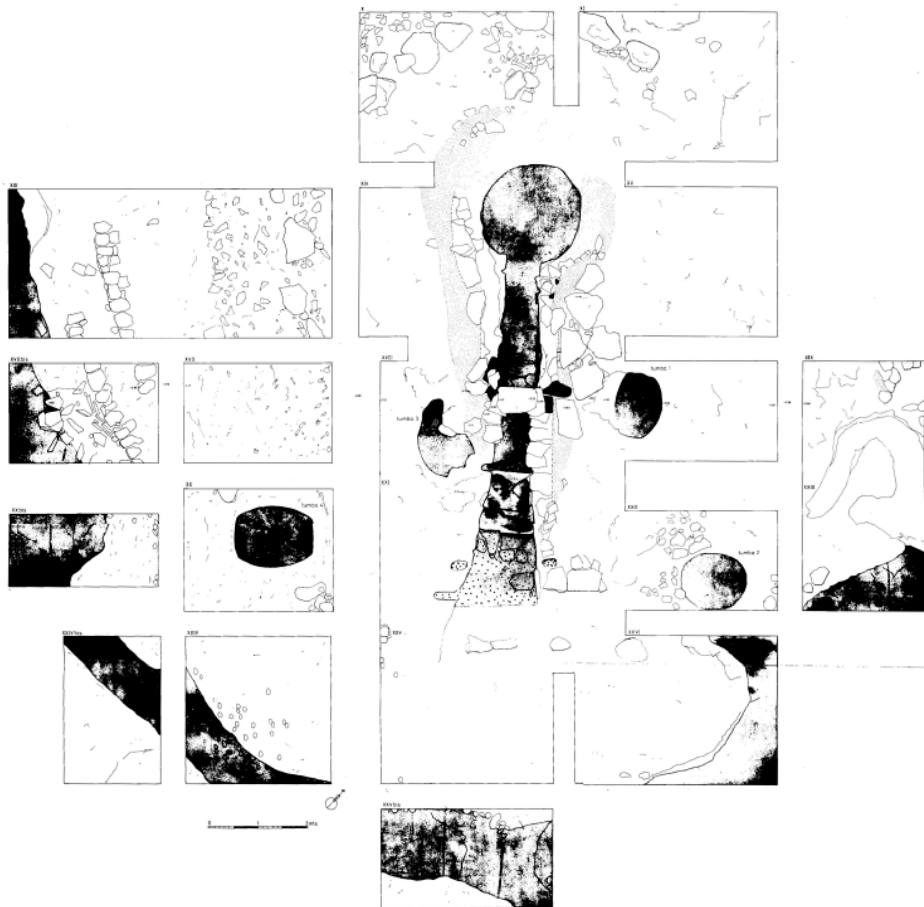
Fig. 3.—Planta de la excavación del Tholos de las Canteras. 1:60.
