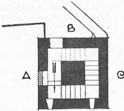
FIG. I.—GRANADA. TORRE DE S. JOSÉ. PLANTA.
