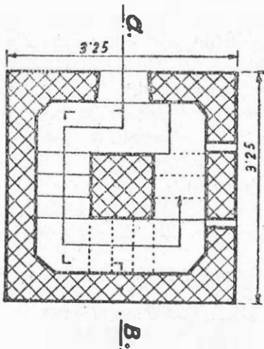
FIG. 7.—BOLLULLOS DE LA MITACIÓN (SEVILLA). ERMITA DE CUATROHABITAN. PLANTA BAJA DEL ALMINAR.
